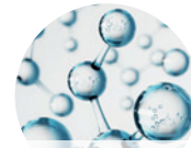
Д-пантенол
