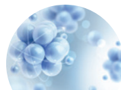
аминокислоты
