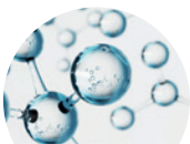
Д-пантенол
