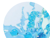
молекулы Volume-up
