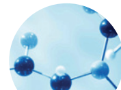
гидролизированный кератин
