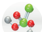
аминокислотный комплекс
