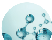
трехалоза
