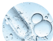
биомиметический пептид
